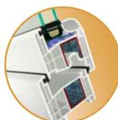
Sistema de 6 cámaras hoja no alineada
